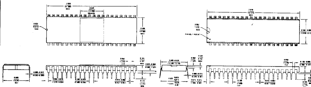
40-Lead Ceramic Dual-in-Line Package (D) Order Number INS8080AD
