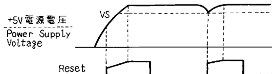
[Fig. 2] PST519 を用いたパワー・オンディレイ回路/Power-ON delay circuit
