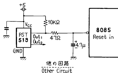
[Fig. 3] 8085 の Reset 回路/Reset circuit of 8085
