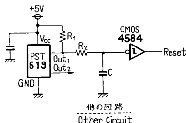
〔第4図〕RESET 脉冲幅 が最小の動作例
