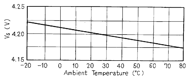
■Vs-温度特性/Vs-Temperature Charac.
