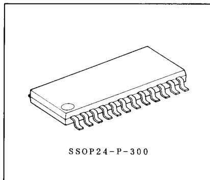
Weight : 0.32g (Typ.)
