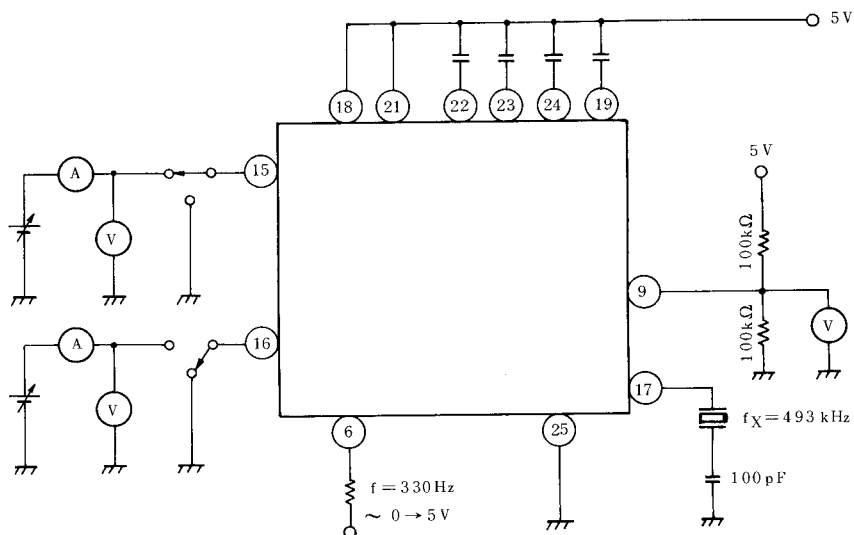
TEST CIRCUIT 5 V_{MS-th} , I_{MS} , V_{ST-th} , I_{ST}
