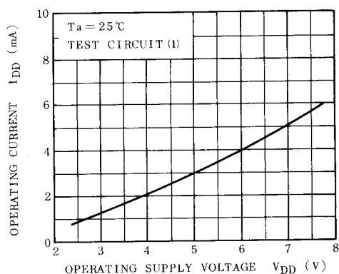
I_{\text{DD}} - V_{\text{DD}}
