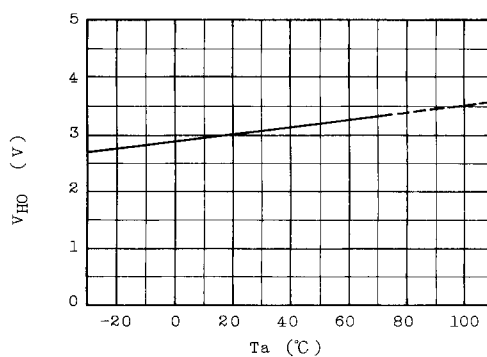
V_{HO} - T_a
