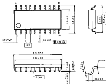
○ SOP 20-P-300A
