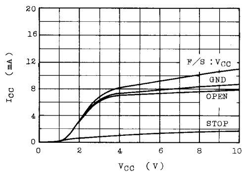
I_{CC} - V_{CC}
