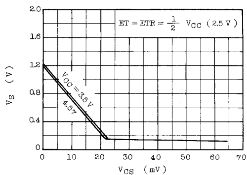
V_S - V_{CS}
