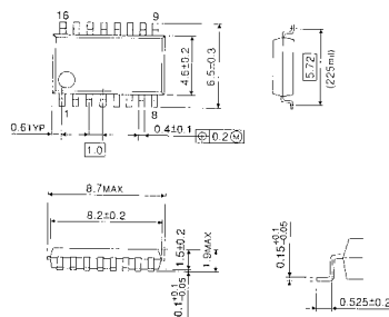
○ SSOP 16 -P-225A
