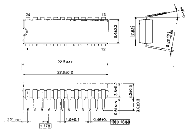
○ SDIP 24-P-300
