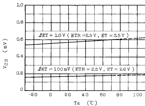
V_{CS} - T_a
