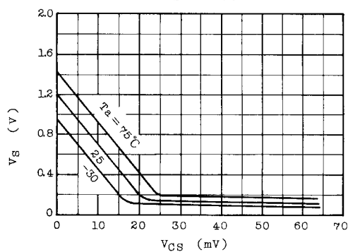
V_S - V_{CS}
