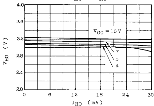
V_{HO} - I_{HO}
