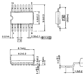
○ SSOP 16-P-300
