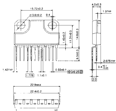
○ HZIP 12-P-B
