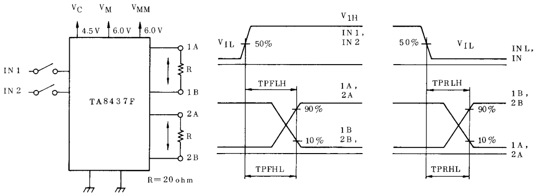
Fig. 3 OUTPUT WAVE
