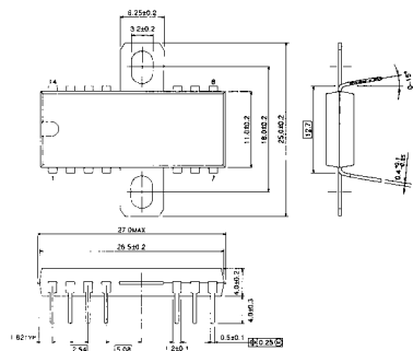
○ HDIP 14-P-500
