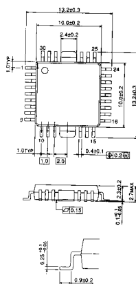
○ HQFP 30-P-1010
