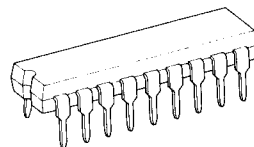
DIP18-P-300D
