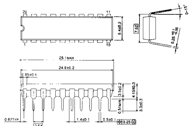
○ DIP 20-P-300A
