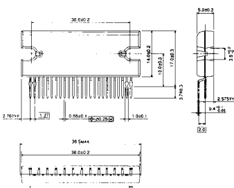
○ HZIP 25-P
