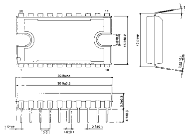
○ HDIP 20-P
