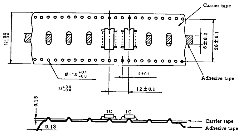
Fig. 6-2 Taping
