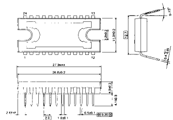
○ HDIP 24-P-500
