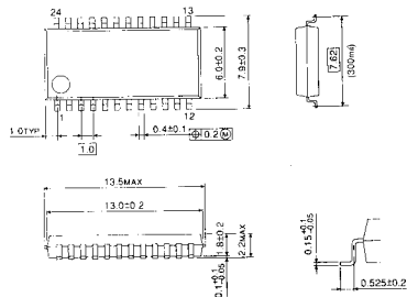
○ SSOP 24-P-300
